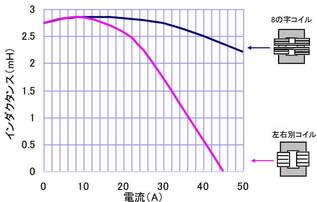
飽和特性代表例
