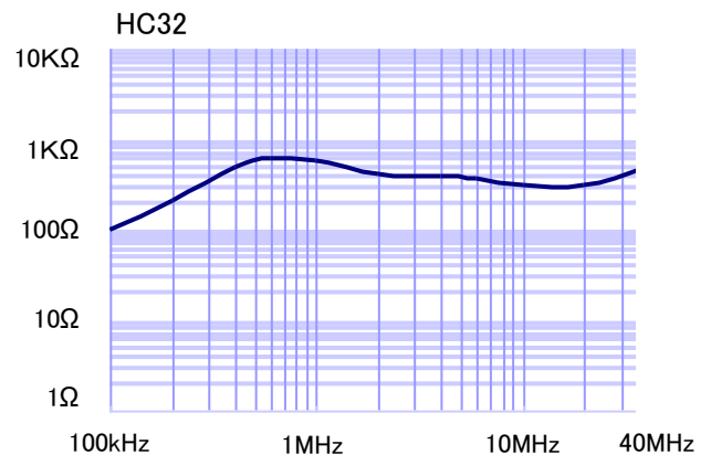
周波数特性(インピーダンス)代表例
