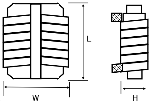
形状(低背タイプ)
